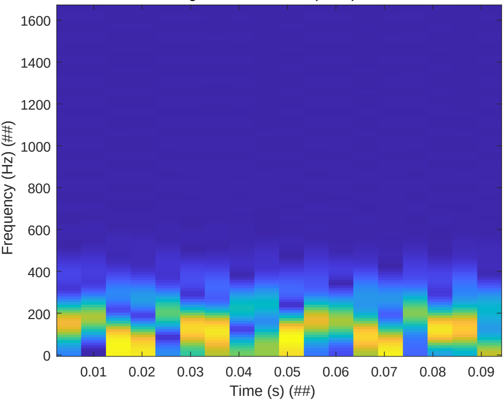
Signal: FM Sinusoid (#####)
